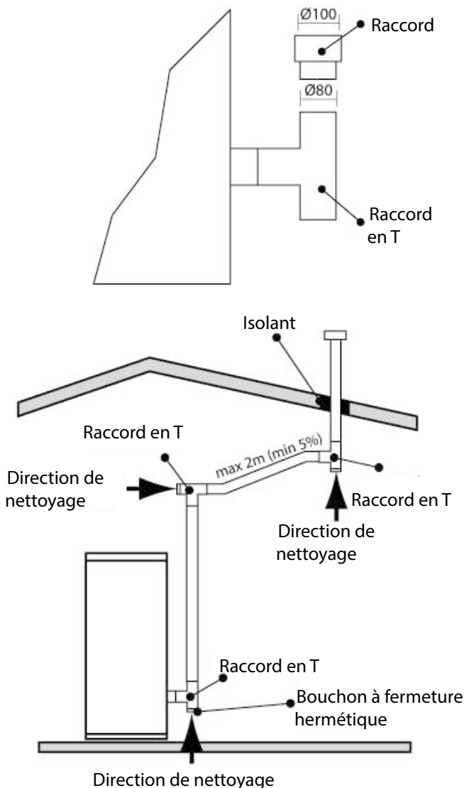
fig. 11 longueurs des tuyaux
