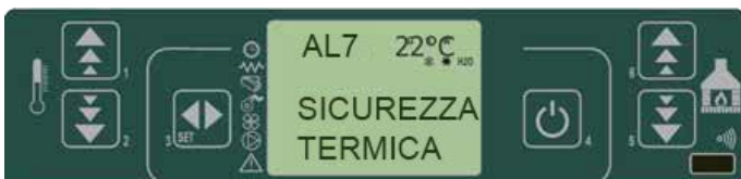
fig. 42 painel de comandos - alarme por termóstato geral
