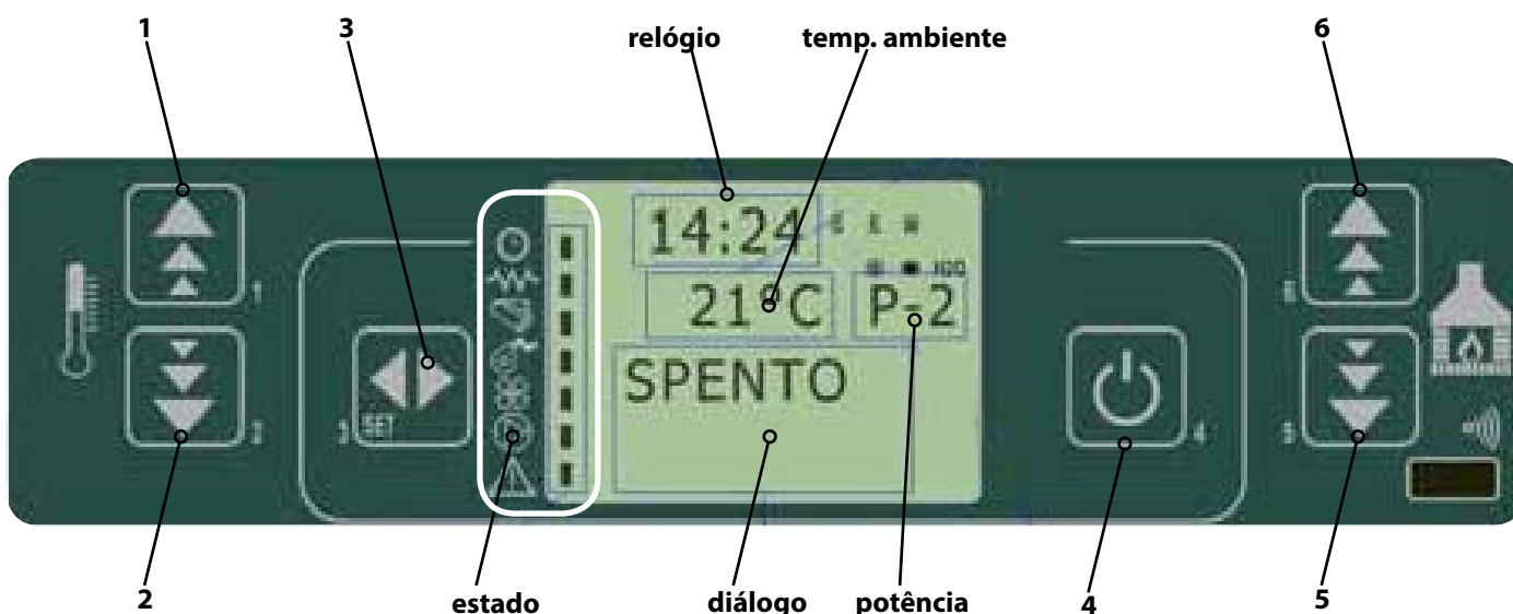
fig. 22 painel de comandos - programação semanal
