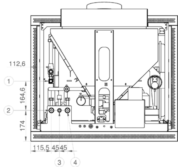
fig. 10 pontos de conexão sem kit sanitário
