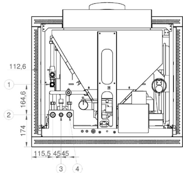
fig. 10 points de raccordement sans kit sanitaire
