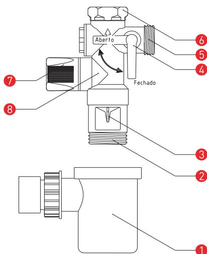
Fig. 3 - Grupo Hidráulico 3/4"
