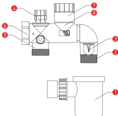
Fig. 4 - Grupo Hidráulico 1"
