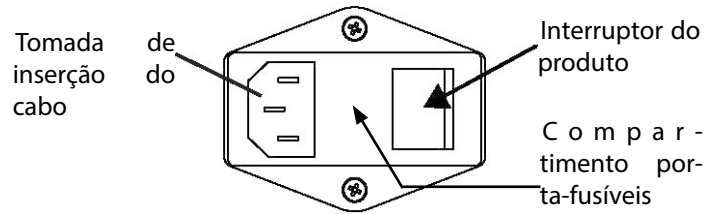
fig. 12 alimentação elétrica
