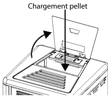
fig. 13 chargement pellet
