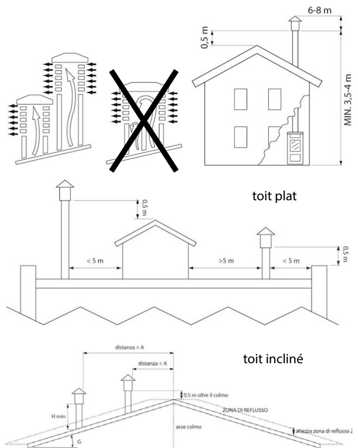
fig. 5 modalités, permises et interdites, d'installation de cheminée
