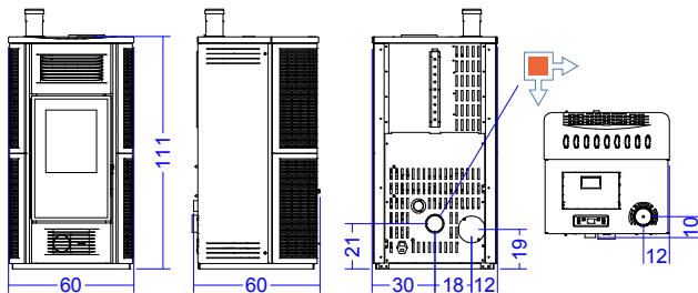
dimensioni di ingombro - overall dimensions - dimensions d'encombrement - dimensiones totales
