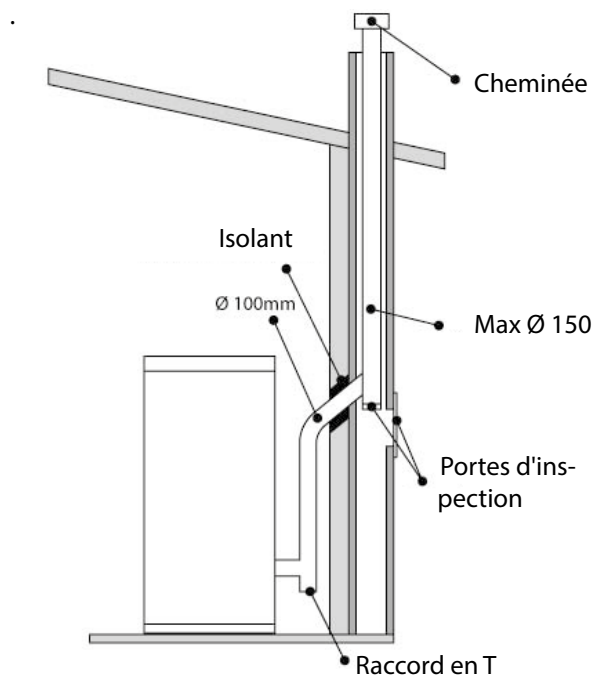
fig. 9 conduit de fumée de type traditionnel
