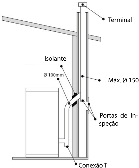
fig. 9 fumeiro de tipo tradicional
