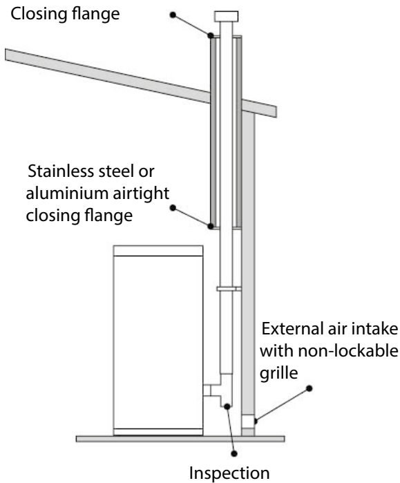
fig. 10 external flue
