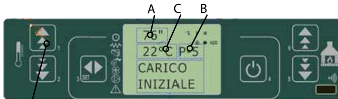
fig. 22 painel de comandos - carregamento de pellets inicial
