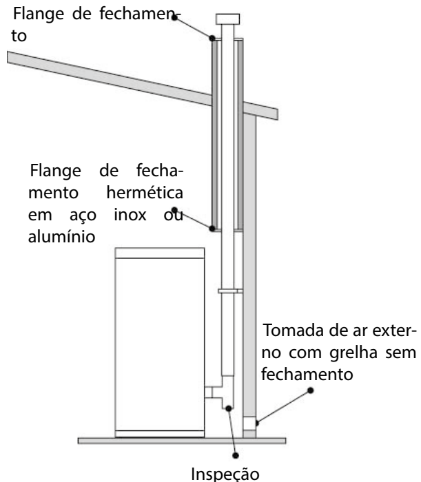
fig. 10 fumeiro tipo externo
