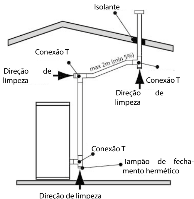
fig. 8 comprimentos dos tubos
