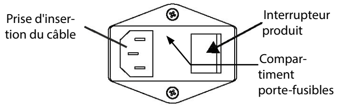
fig. 12 alimentation électrique
