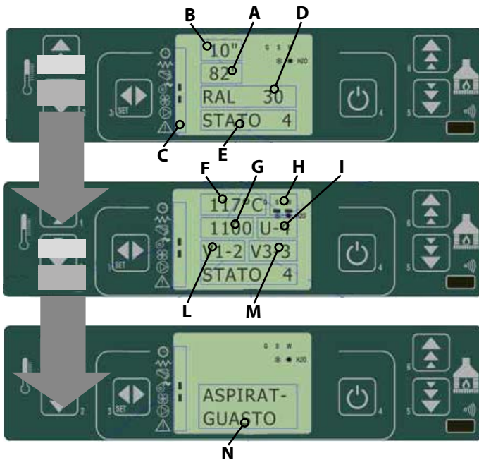
fig. 23 tableau de commande - écran d'état du produit
