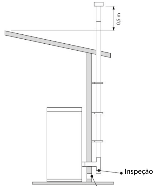
Tomada de ar com grelha sem fechamento -- fig. 10 fumeiro tipo externo
