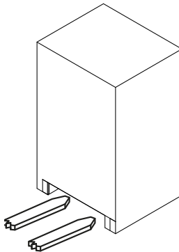
fig. 2 levage emballage
