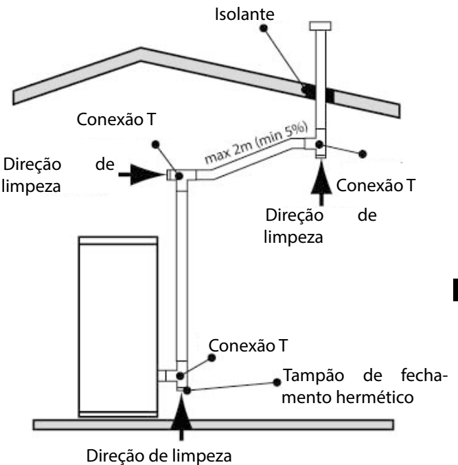
fig. 8 comprimentos dos tubos
