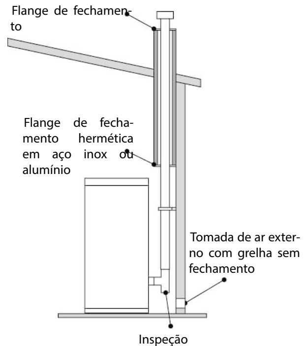
Tomada de ar com grelha sem fechamento -- fig. 10 fumeiro tipo externo
