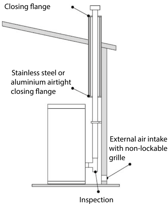
fig. 10 external flue
