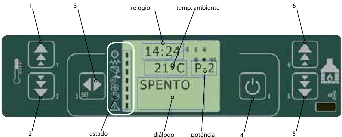
fig. 14a Descrição dos botões
