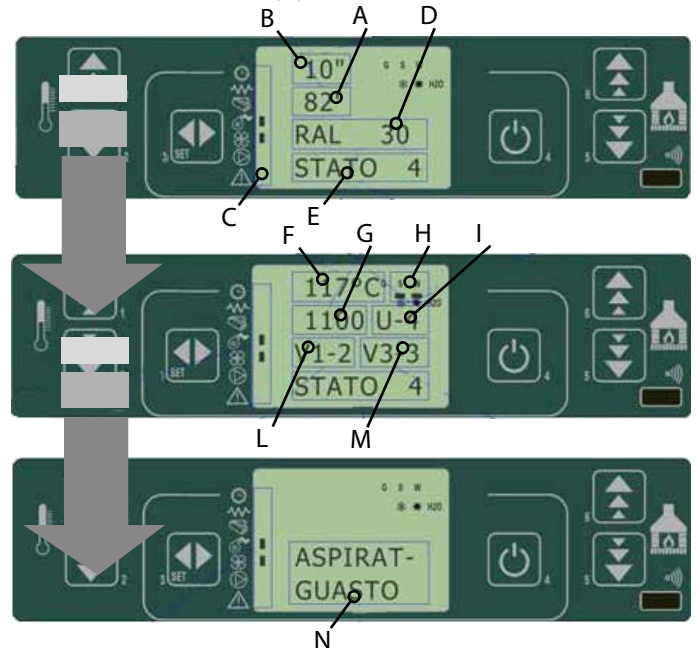
fig. 23 painel de comandos - ecrã de estado do produto
