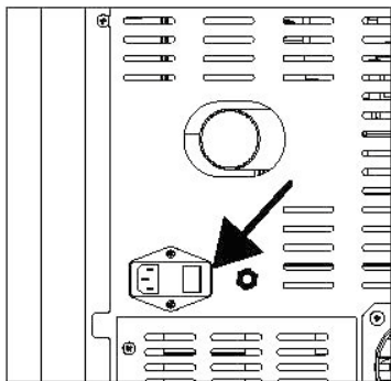
fig. 11 ligação elétrica da estufa
