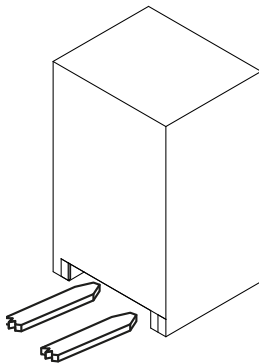
fig. 2 elevação da embalagem
