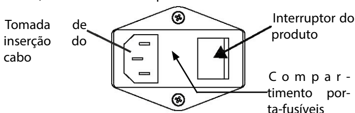
fig. 12 alimentação elétrica
