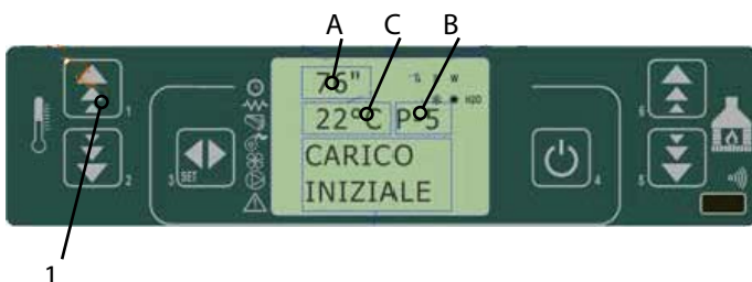
fig. 22 painel de comandos - carregamento de pellets inicial
